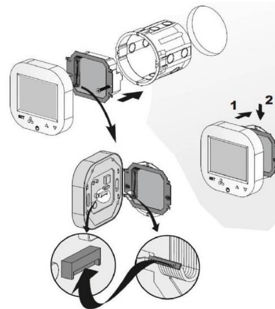
Сборочный чертеж
