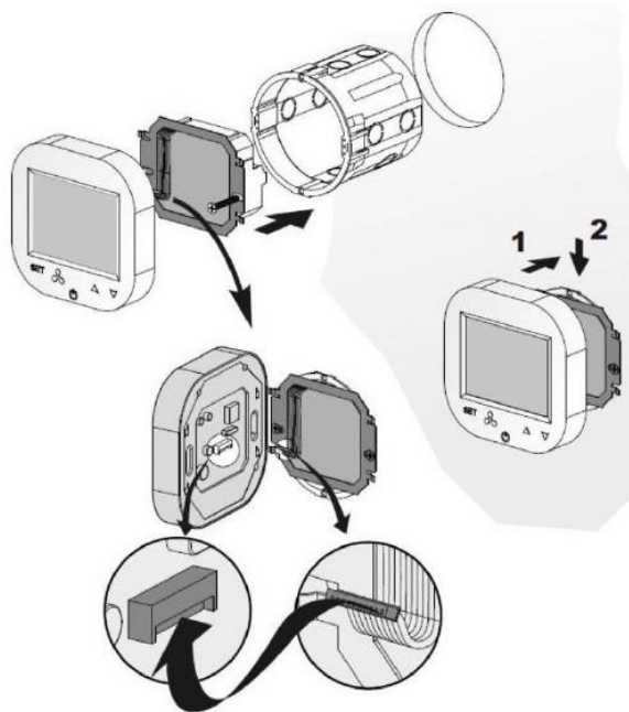
Schemat montażowy
