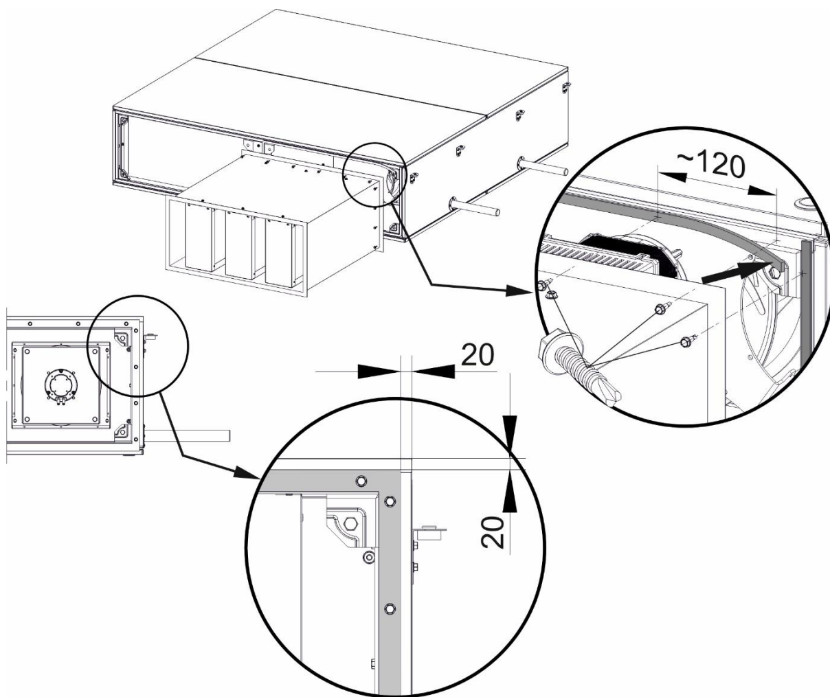
Rys. 8c. Łączenie sekcji tłumików do sekcji bazowej
