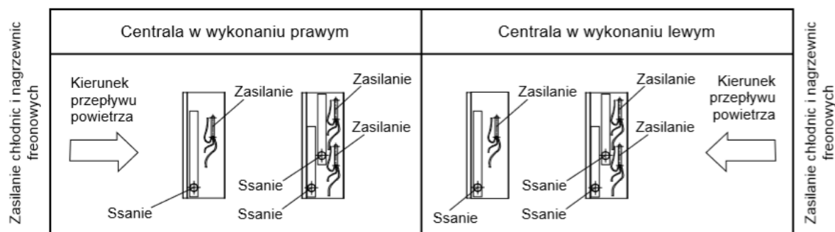
Rysunek 13 Zasilenie chłodziw freonowych oraz nagrzewnic
