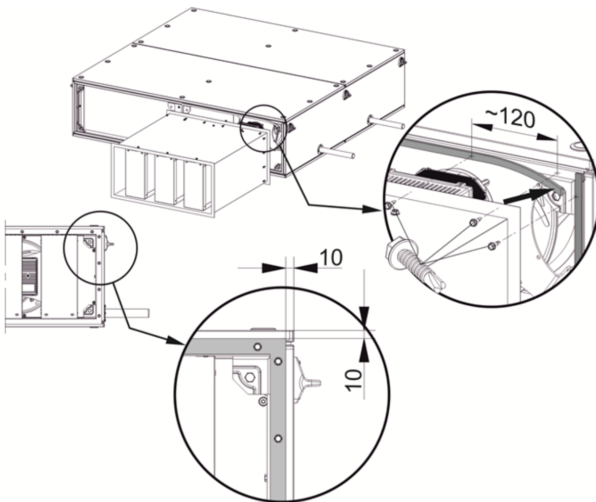
Rys. 8c. Łączenie sekcji tłumików do sekcji bazowej
