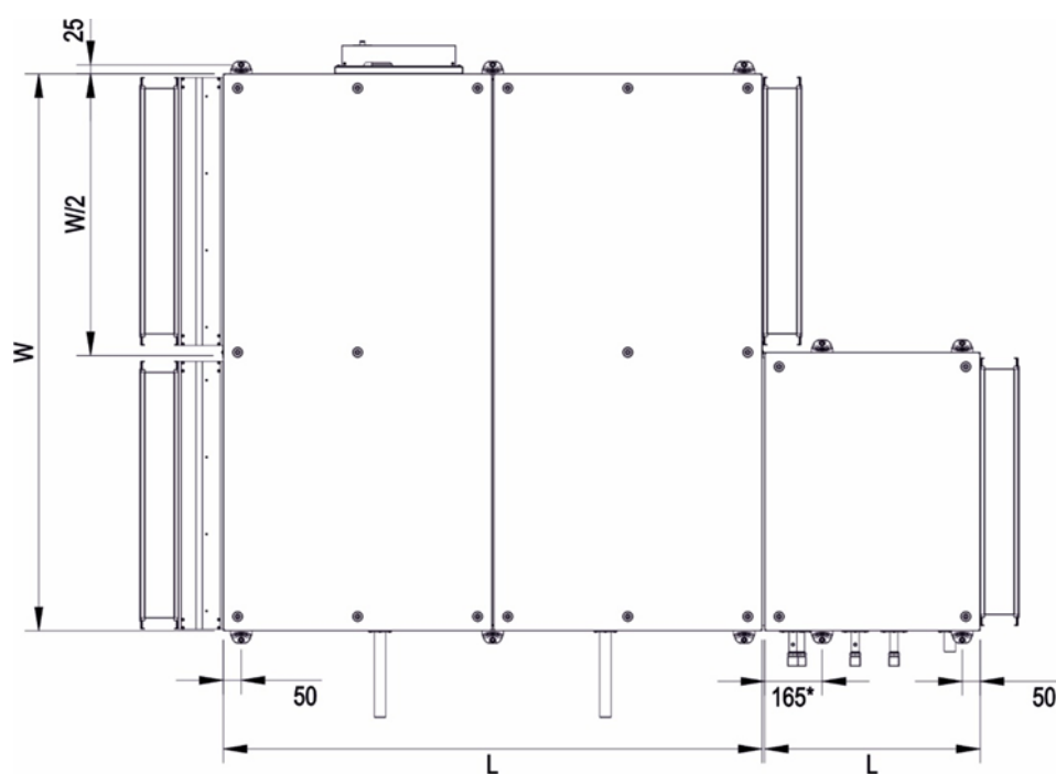
Rys. 7. Konfiguracja uchwytów do zawieszenia.
