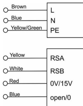
Rys.20 Połączenie kablowe silnika z wentylatorem dla urządzenia VVS005s
