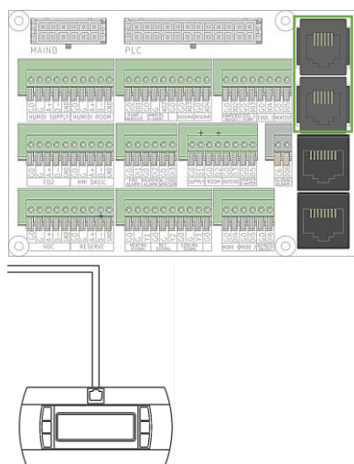
Podłączenie terminala – HMI Advance (N3)
