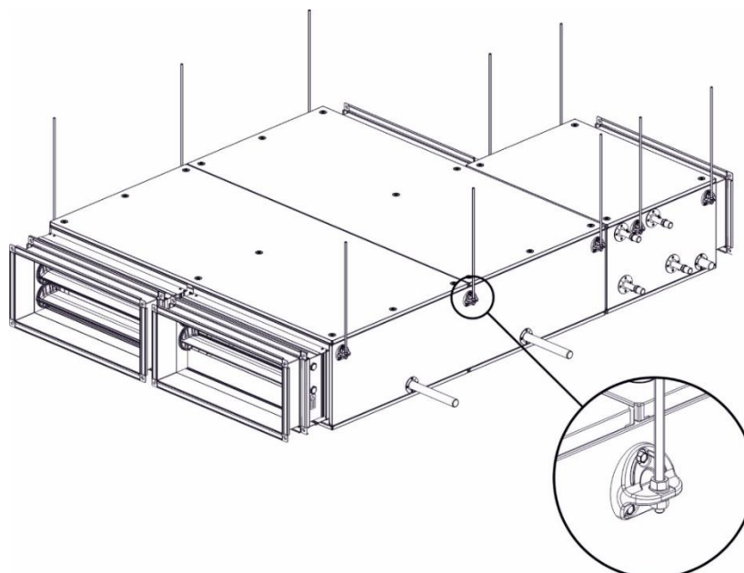
Rys.6b. Przykład zawieszenia sekcji centrali.
