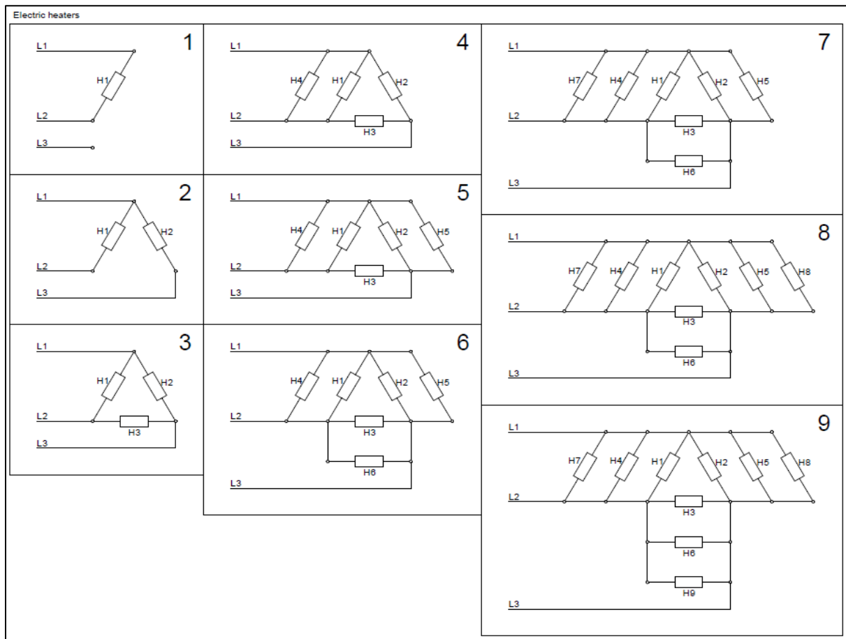
Rys 18 Schematy połączeń dla grzałek elektrycznych
