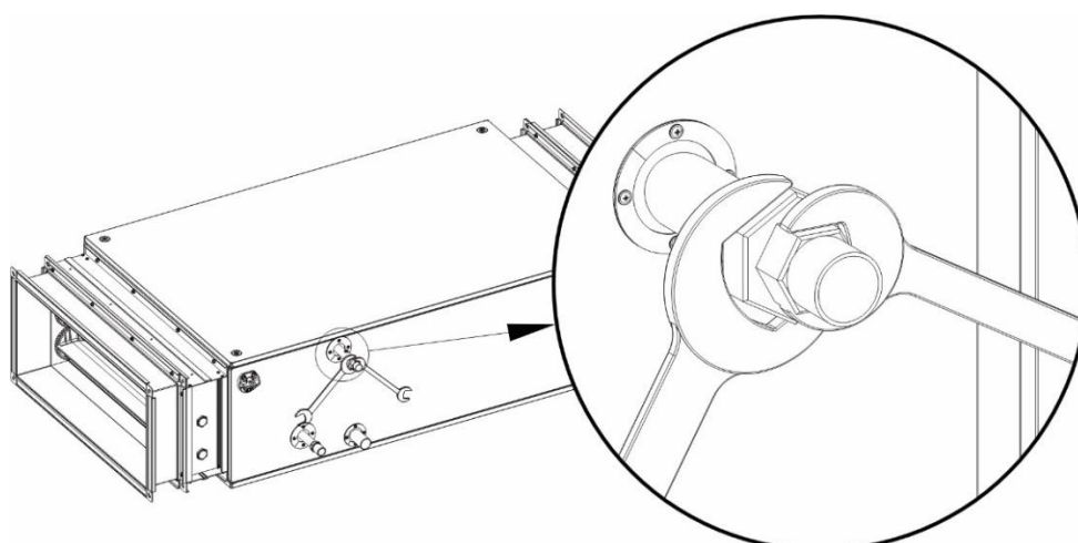
Rys.11. Zabezpieczenie skręconych połączeń wymiennika.
