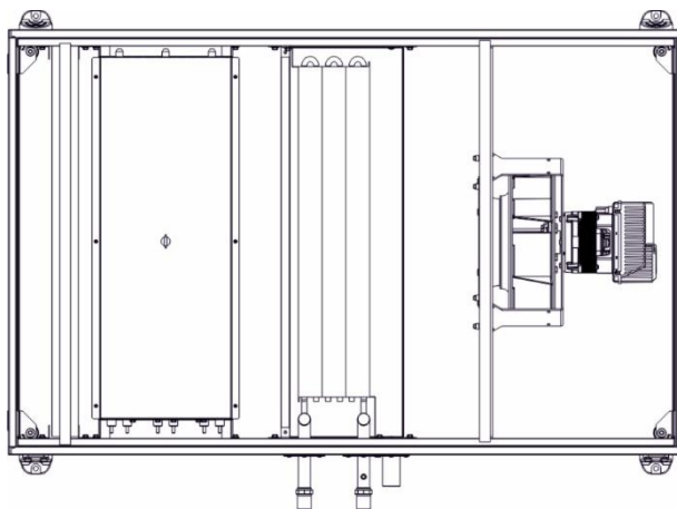
Rys. 4. Przykłady sekcji.
