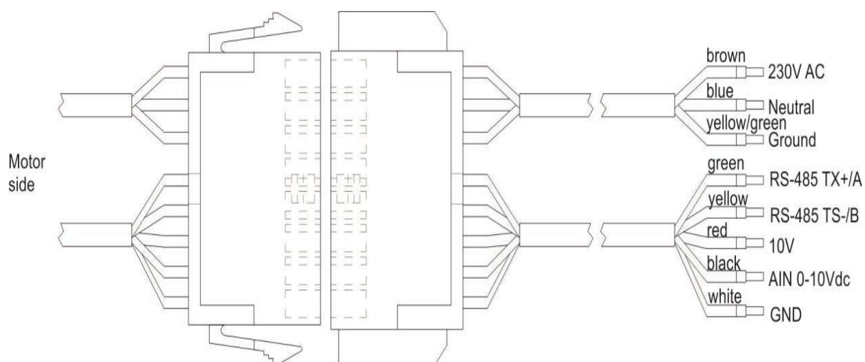
Rys.21. Wiązka kablowa silników central VVS010-VVS030
