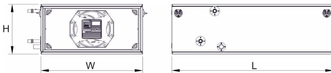
Rys.5. Wymiary sekcji.
