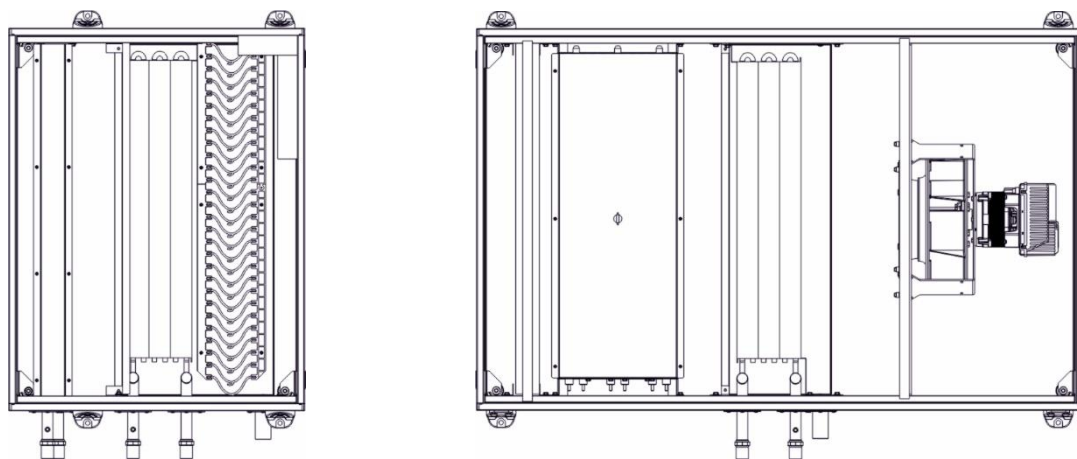
Rys. 4. Przykłady sekcji.
