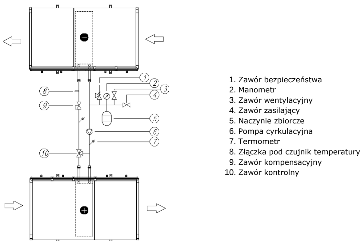
Rys.14. Przykłady podłączania wymienników do instalacji zasilających
