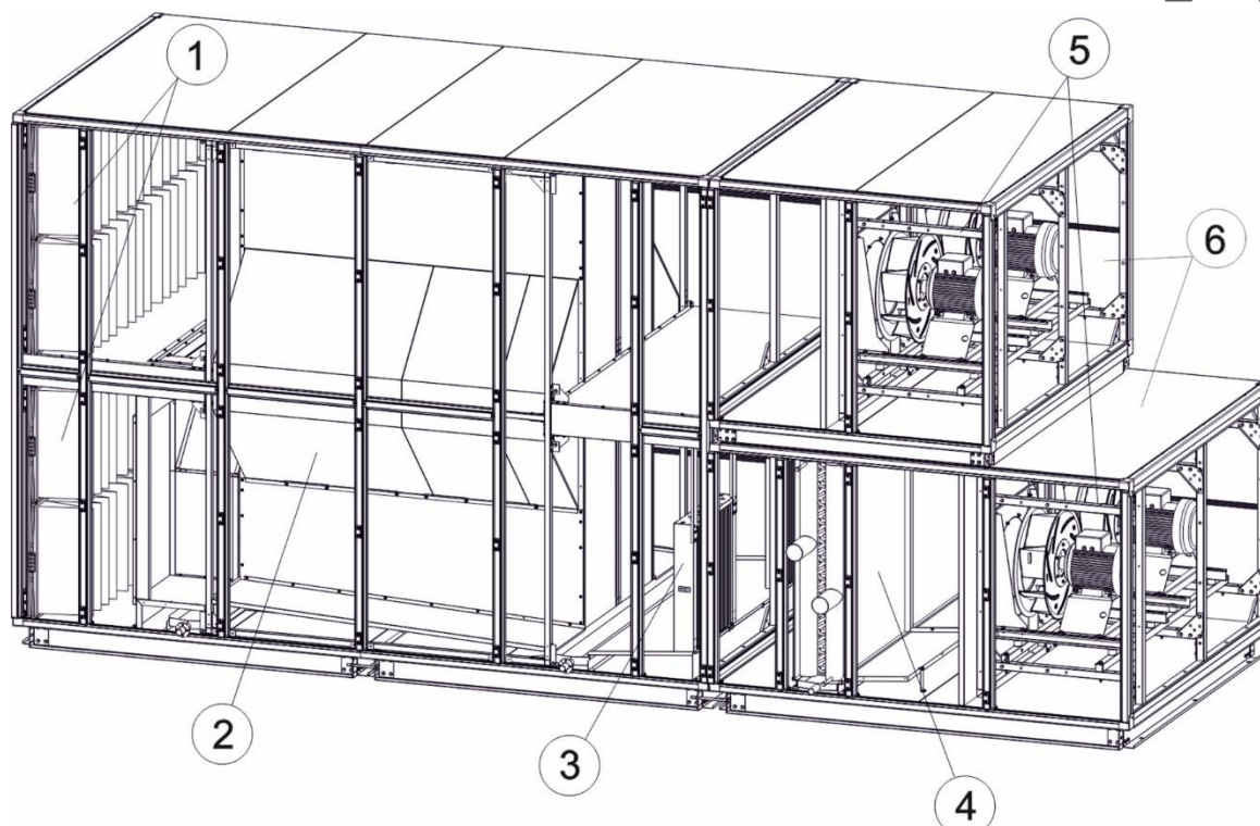
Rys.3. Przykład urządzenia nawiewno-wyiewnego: 1 – filtr kieszeniowy, 2- wymiennik heksagonalny, 3 - odkraplacz, 4 – chłodnica, 5 – zespoły wentylatorowe, 6 – obudowa
