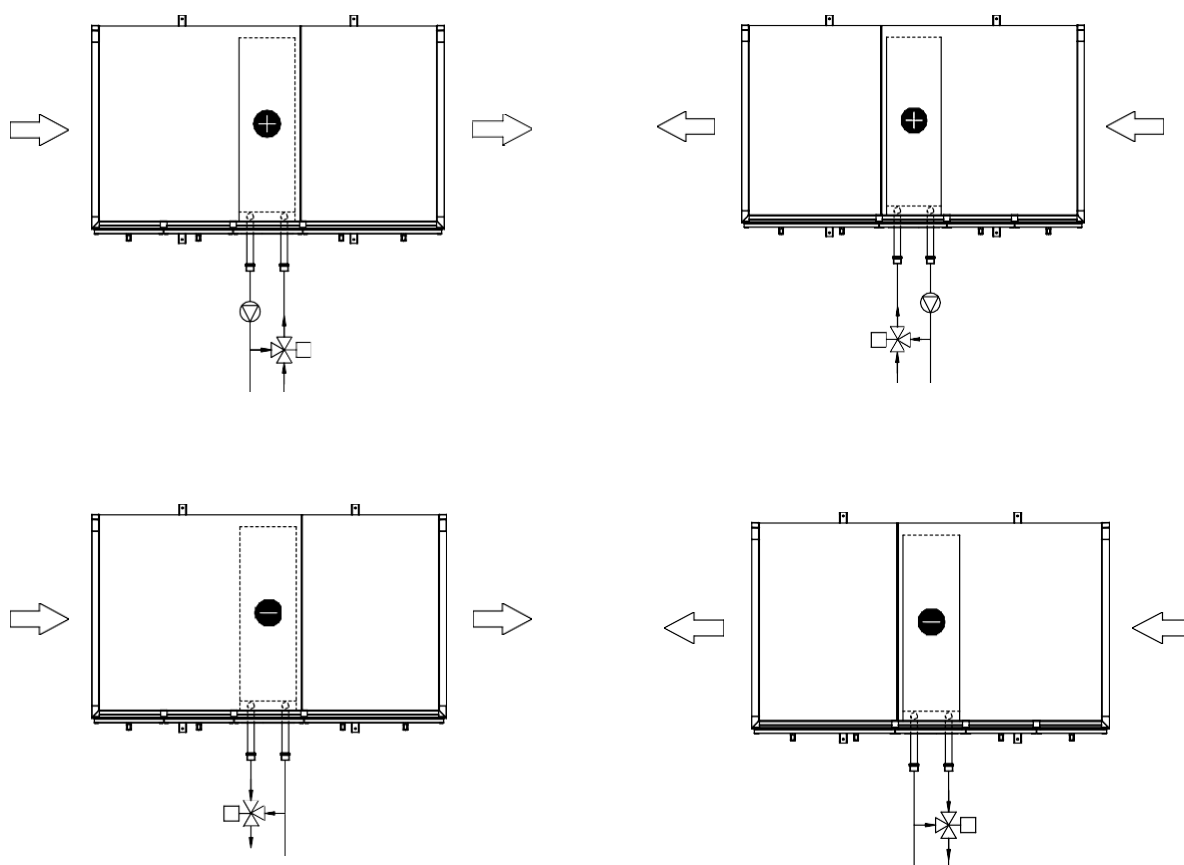
Rys.12. Przykłady zasilania wymienników wodnych
