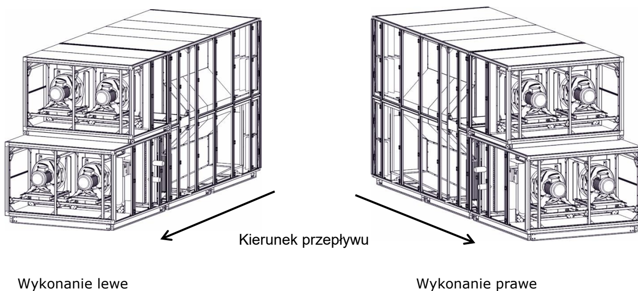
Rys. 4 Wersja VS 21-650
