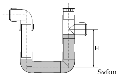
Rys.16. Typy syfonów
