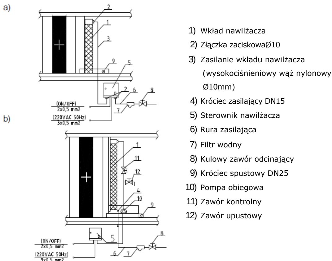
Rys.15. Nawilżacz złożowy
