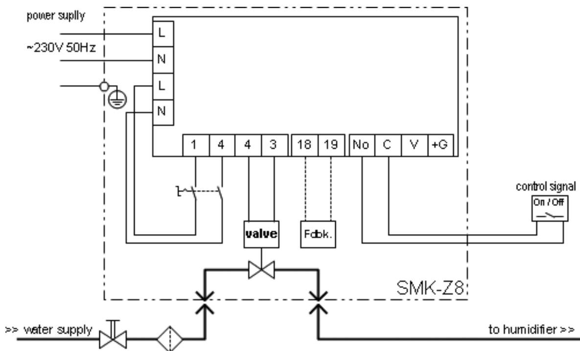
Rys.17.a. Schemat podłączenia nawilzacza z bezpośrednim zasilaniem wodą
