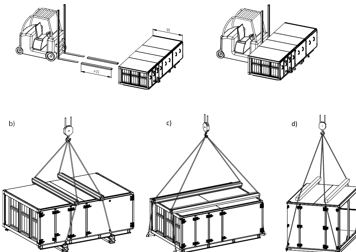
Rys.5. Transport za pomocą dźwigu
