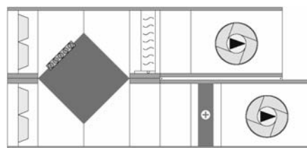
Centrala z wymiennikiem krzyżowym
