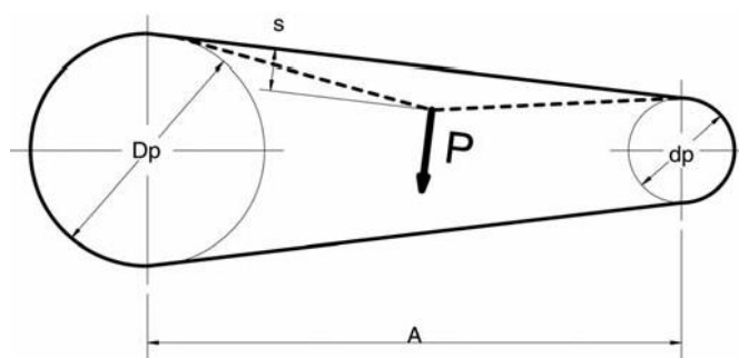
Rys.24 Ugięcie pasa klinowego
