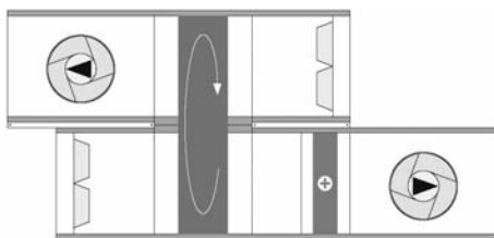
Centrala z wymiennikiem obrotowym
