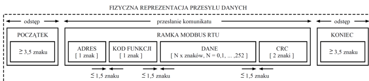
Рис. 7. Передача данных в стандарте MODBUS RTU реализована в преобразователе.
