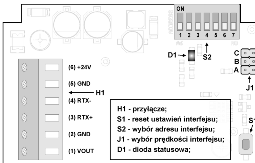
Рис. 2. Описание терминала преобразователя в версии воздуховода : H1 - соединительные контакты; S1 - сброс настроек интерфейса; S2 - настройка адреса интерфейса; J1 - настройка скорости интерфейса; D1 - диод состояния.
