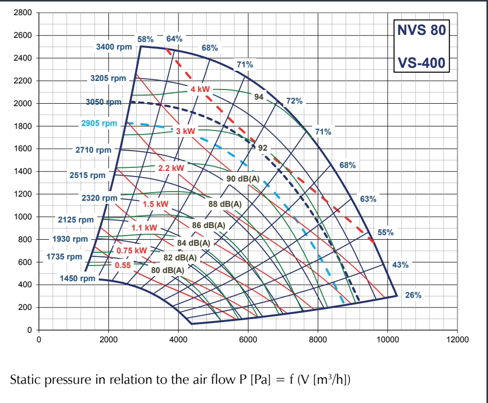
Fan performance NVS 80
