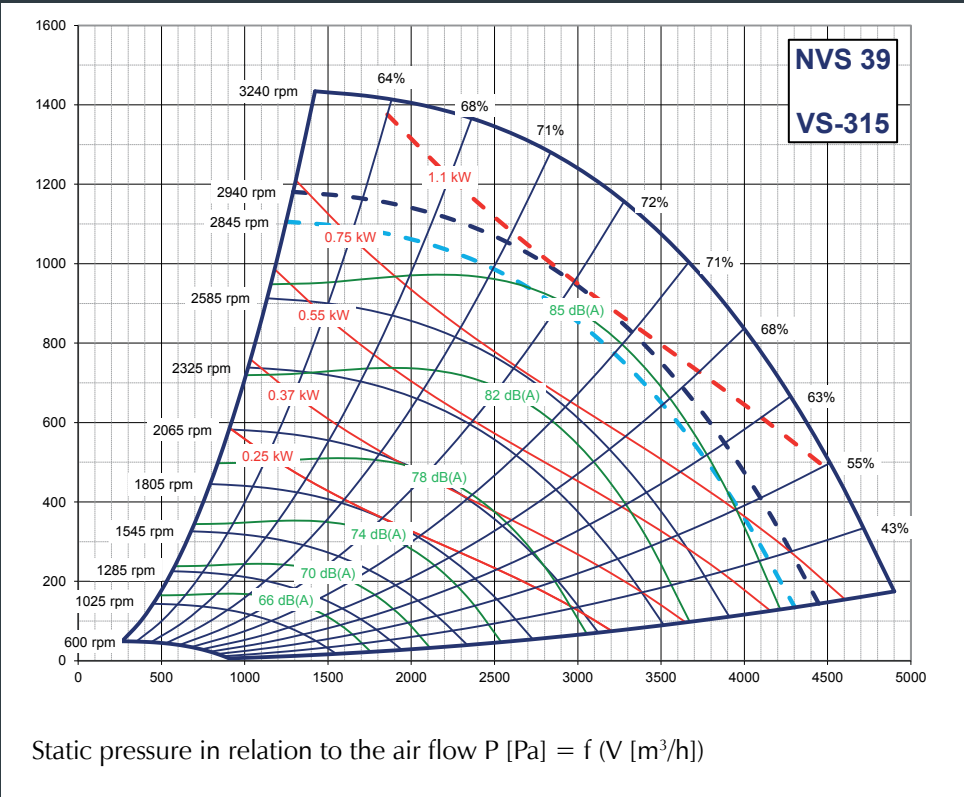
Fan performance NVS 39
