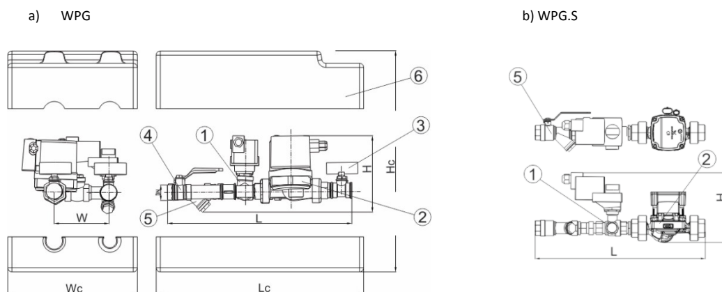
Rys.1. Struktura węzła
