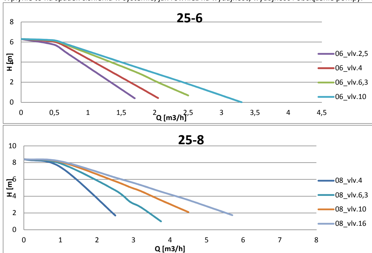
Rys.3. Charakterystyka pomp
