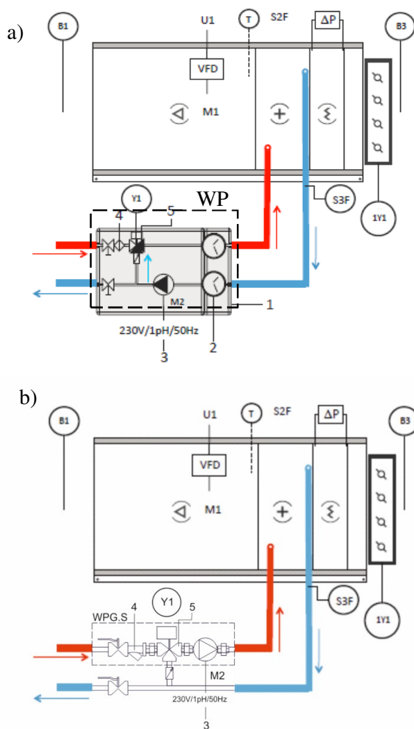
Rys.2. Schemat działania z pełnym WPG (a) i prostym WPG.S (b)
