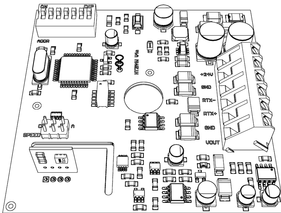
Rysunek 1. Widok obwodu drukowanego wersji naściennej przetwornika.
