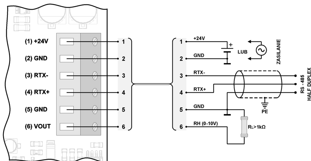
Rysunek 3. Schemat podłączenia przetwornika w wersji naściennej .
