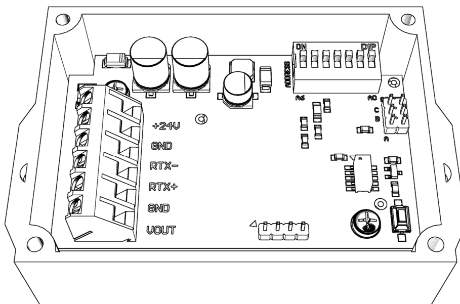
Rysunek 1. Widok obwodu drukowanego wersji naścienniej przetwornika.
