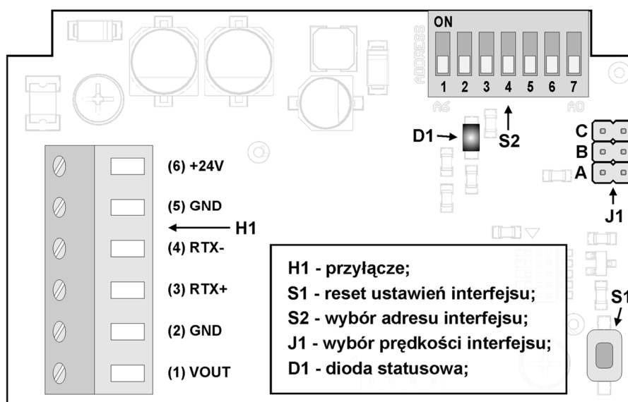
Rysunek 2. Opis wyprowadzeń przetwornika w wersji naściennej .
